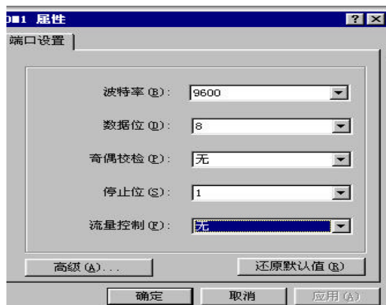
图 5.3 设置超级终端时的串口参数
