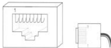
图2.9 网络接口形状以及引脚顺序
