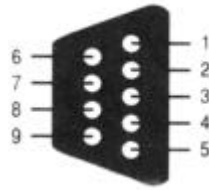
图2.6 SD565设备的操作维护接口形状以及引脚顺序
