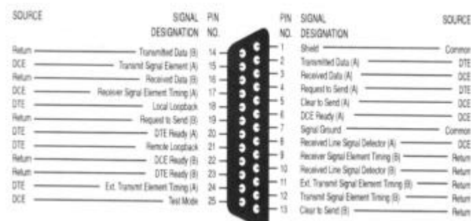
图2.8 SD560同步接口形状以及对应的信号
