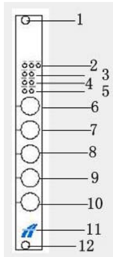
图2.2 SD560LIU模块各个组成部分
