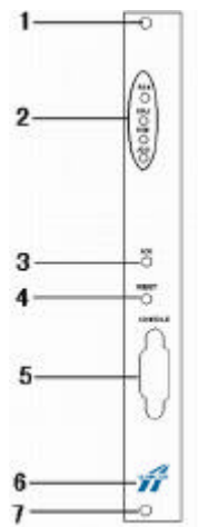
图 2.1 SD560MCU 模块面板以及各部分划分
