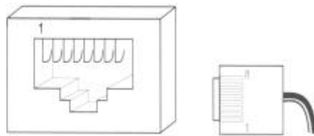
图2.7 SD560异步接口形状以及引脚信号顺序
