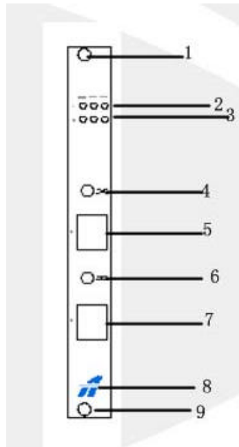
图 2.3 SD560LAN 模块组成
