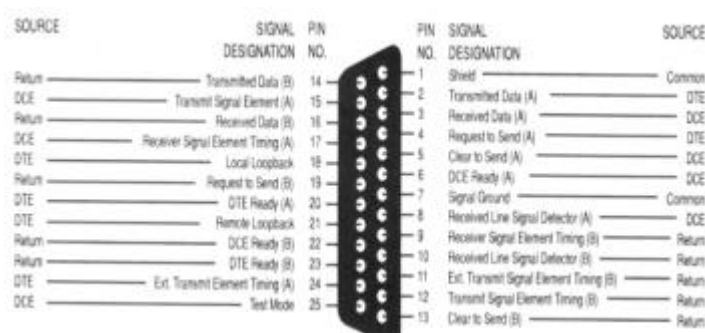
图2.10 SD530同步接口形状以及对应的信号
