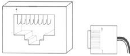
图2.9 SD530异步接口形状以及引脚信号顺序
