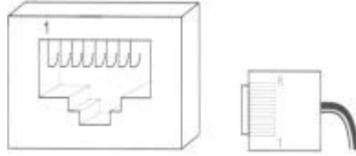
图 2.11 网络接口形状以及引脚顺序
