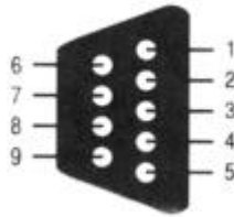
图2.8 SD530复接系统的操作维护接口形状以及引脚顺序
