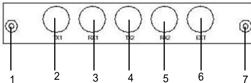
图2.4 LIU模块的组成
